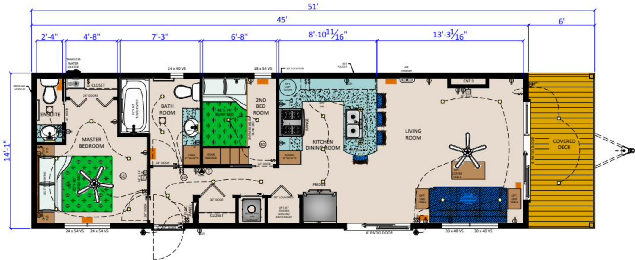
PADDINGTON - 26 (P5114 2BR) (634 SQ.FT.) STANDARD CSA-Z240MH
