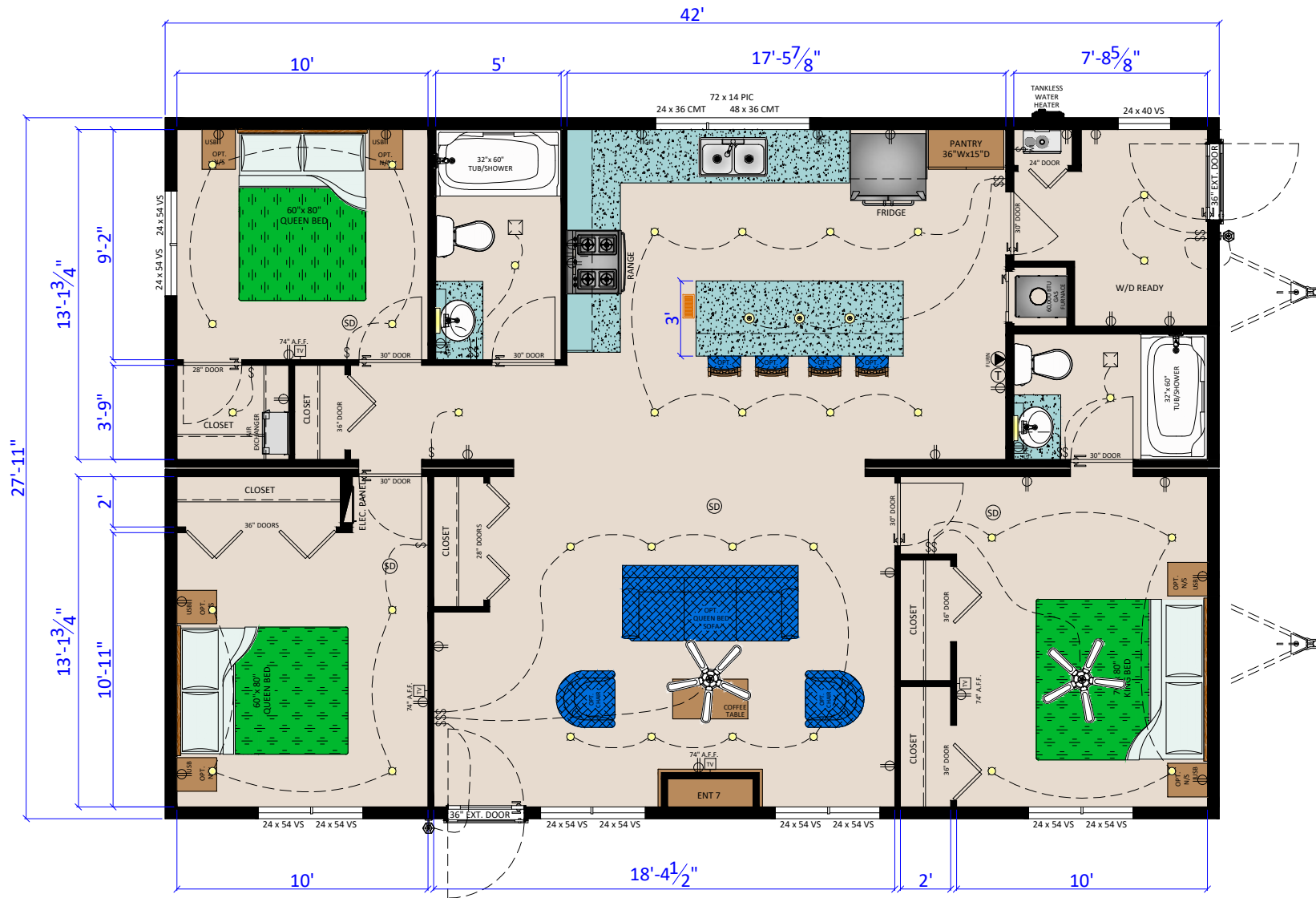
PALGRAVE - 26 (P4214 3 BR) (1172.5 SQ.FT.) STANDARD CSA-Z240MH
