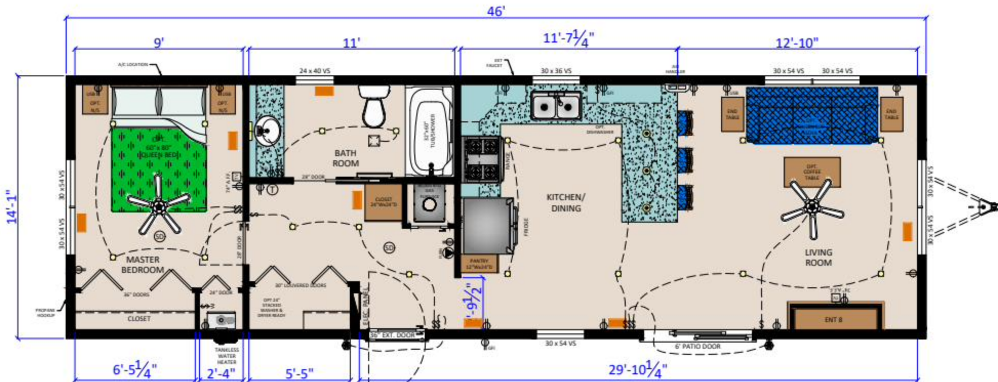
PARKDALE - 26 (P4614 1BR) (647.8 SQ.FT.) STANDARD CSA-Z240MH
