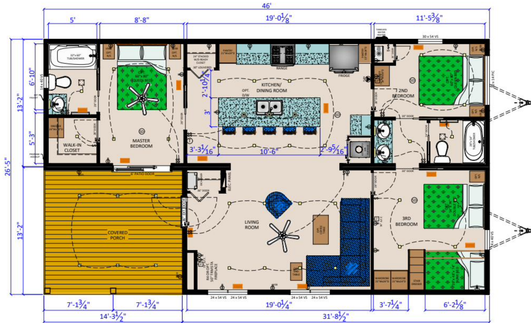
PONOKA - 26 (P4626 3 BR) (1023.1 SQ.FT.) STANDARD CSA-Z240MH
