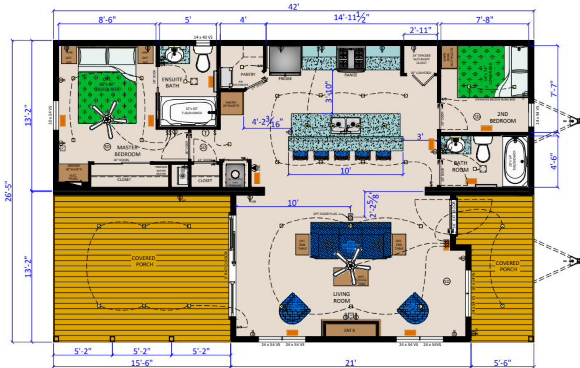
PORTREE - 26 (P4226 2 BR) (823.3 SQ.FT.) STANDARD CSA-Z240MH
