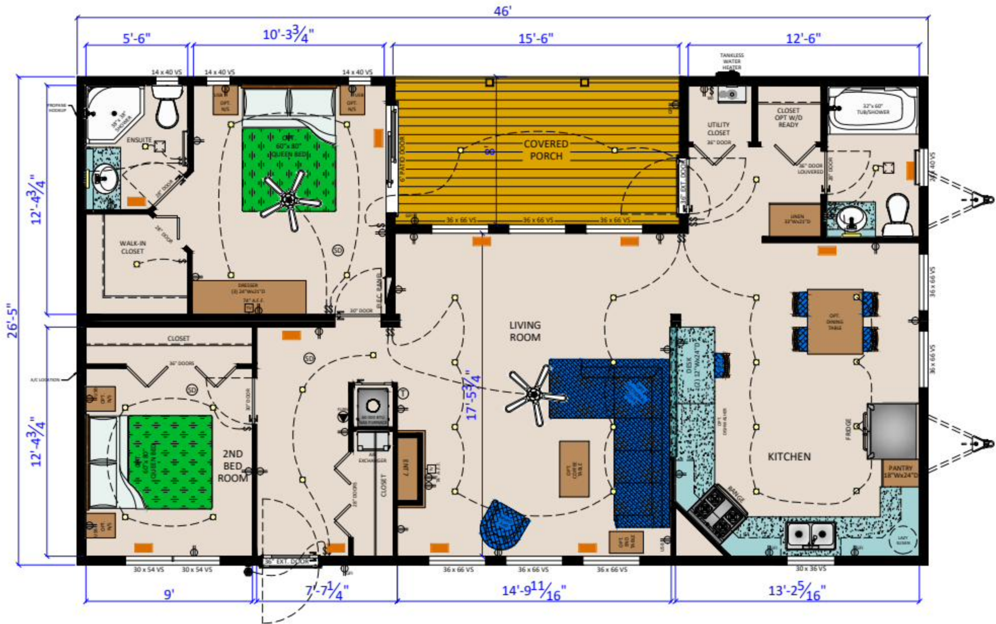
PRISTINA - 26 (P4626 2BR) (1046.3 SQ.FT.) STANDARD CSA-Z240MH
